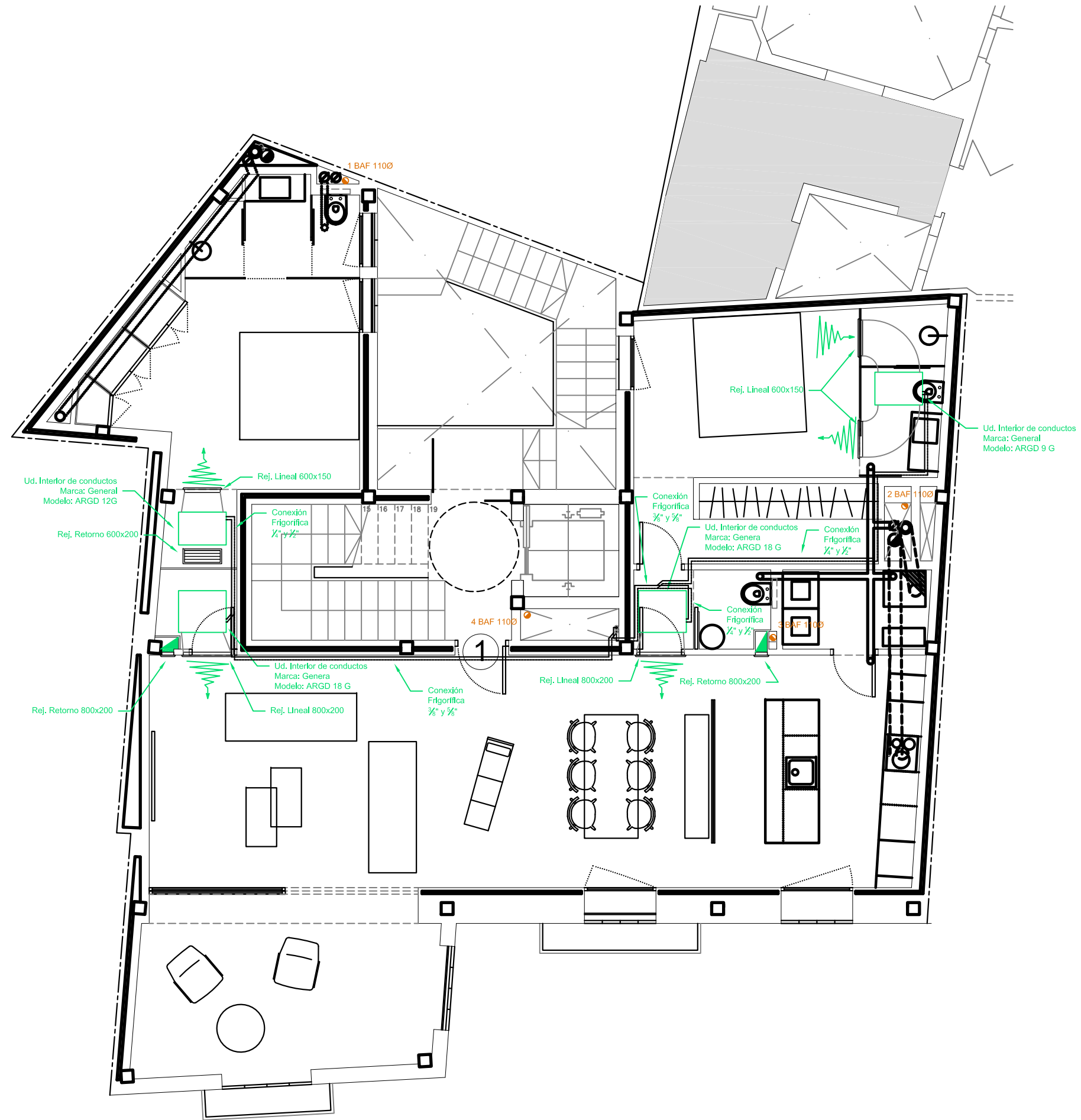
EDIFICIO 1 - PLANTAS PISO 1, 2 y 3 SUPERFICIE CONSTRUIDA 156.88 m2 EDIFICIO 2 - PLANTAS PISO 1, 2 y 3 SUPERFICIE CONSTRUIDA 14.11 m2
