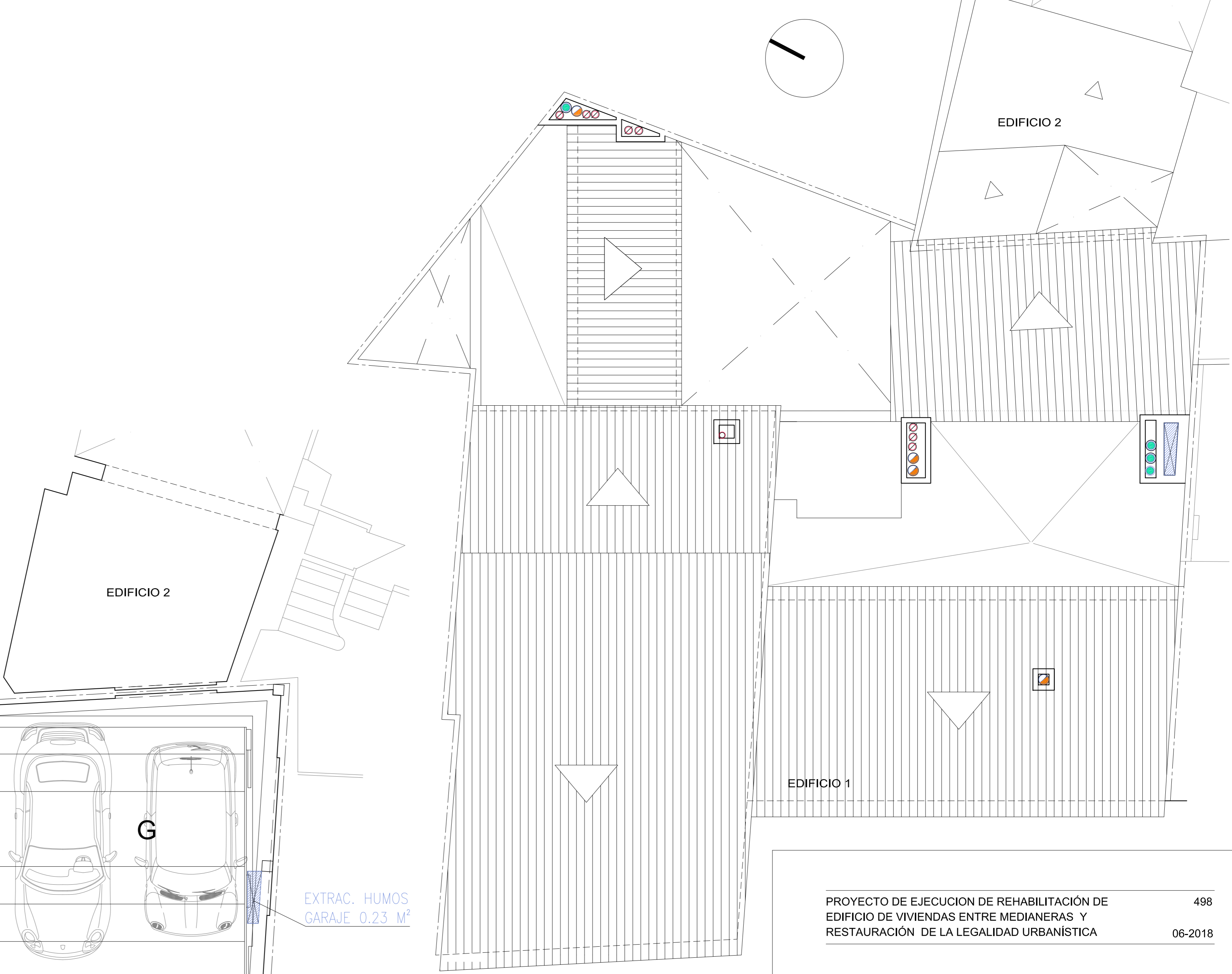
PLANTA CUBIERTA
