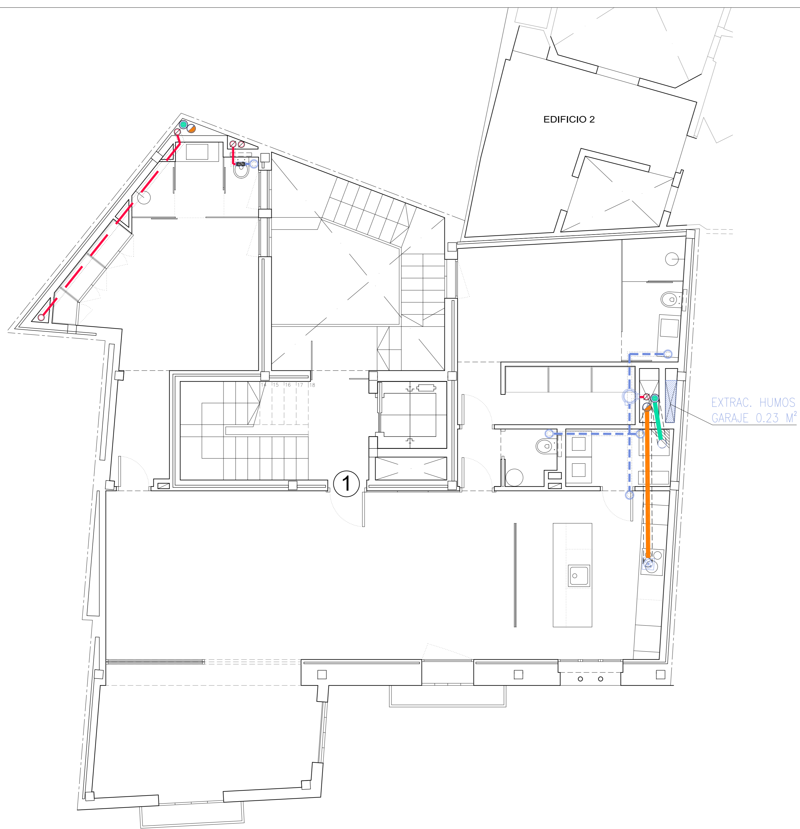
EDIFICIO 1 - PLANTA PISO 1
