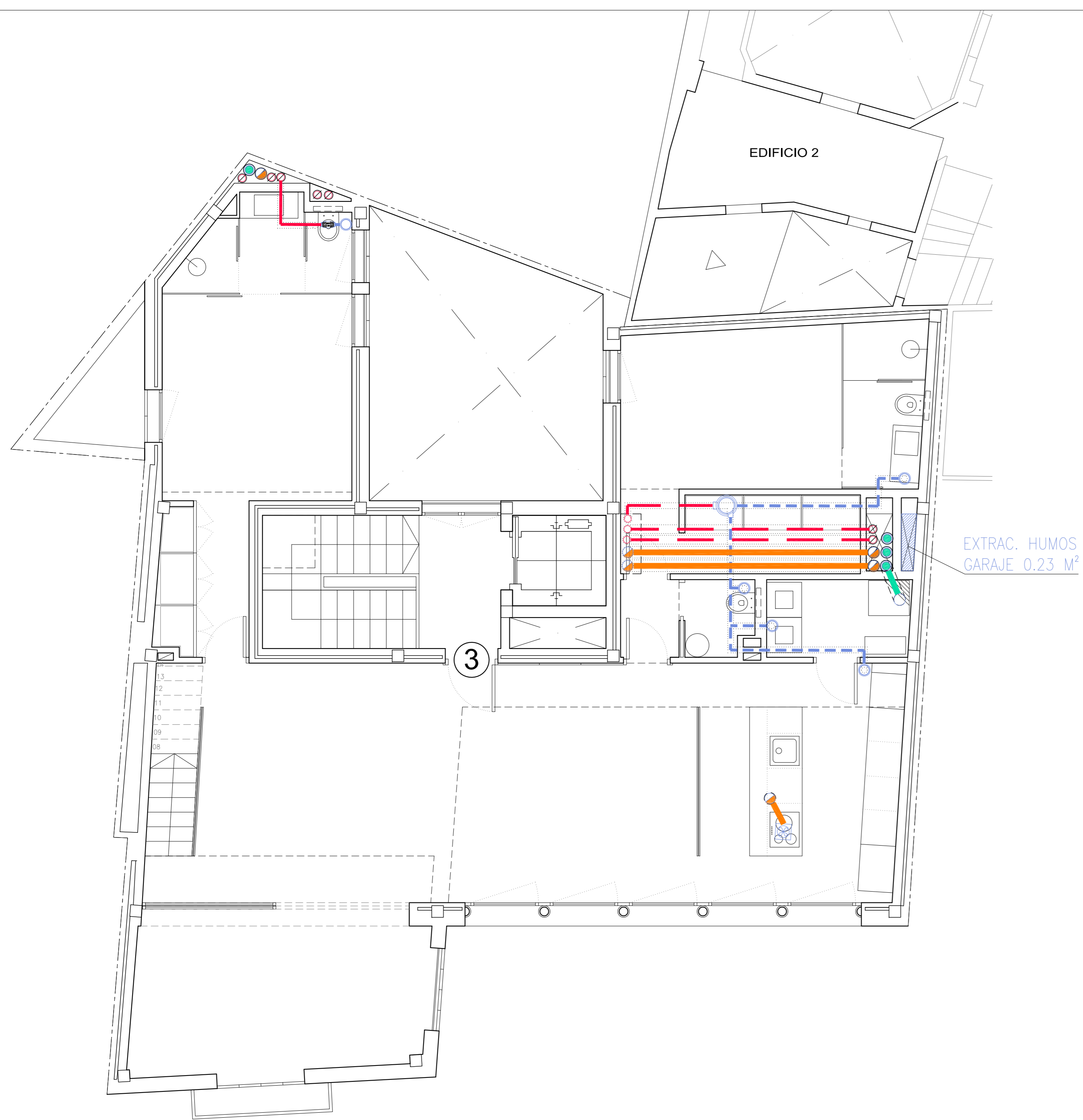
EDIFICIO 1_PLANTA PISO 3
