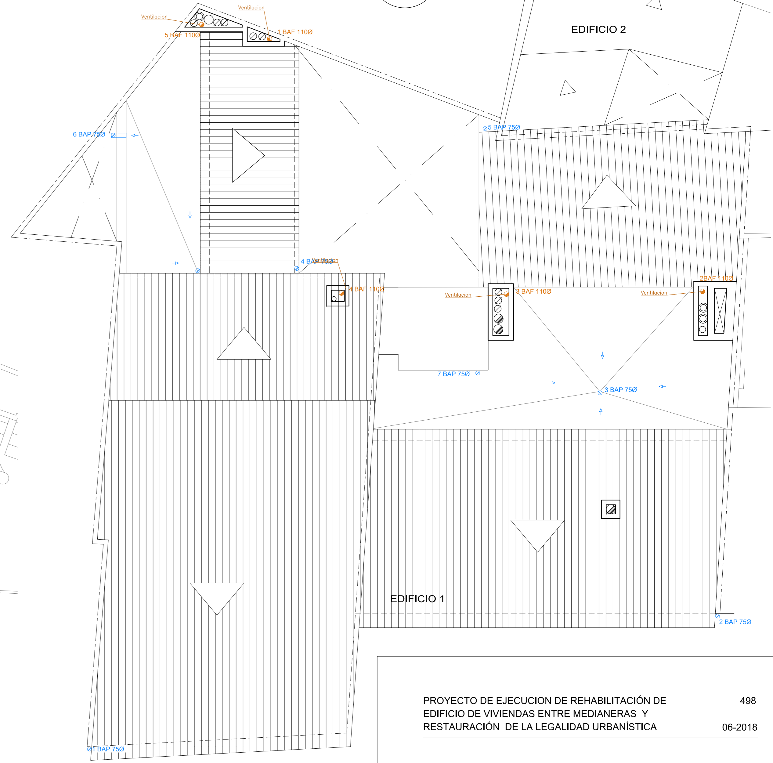
PLANTA CUBIERTA
