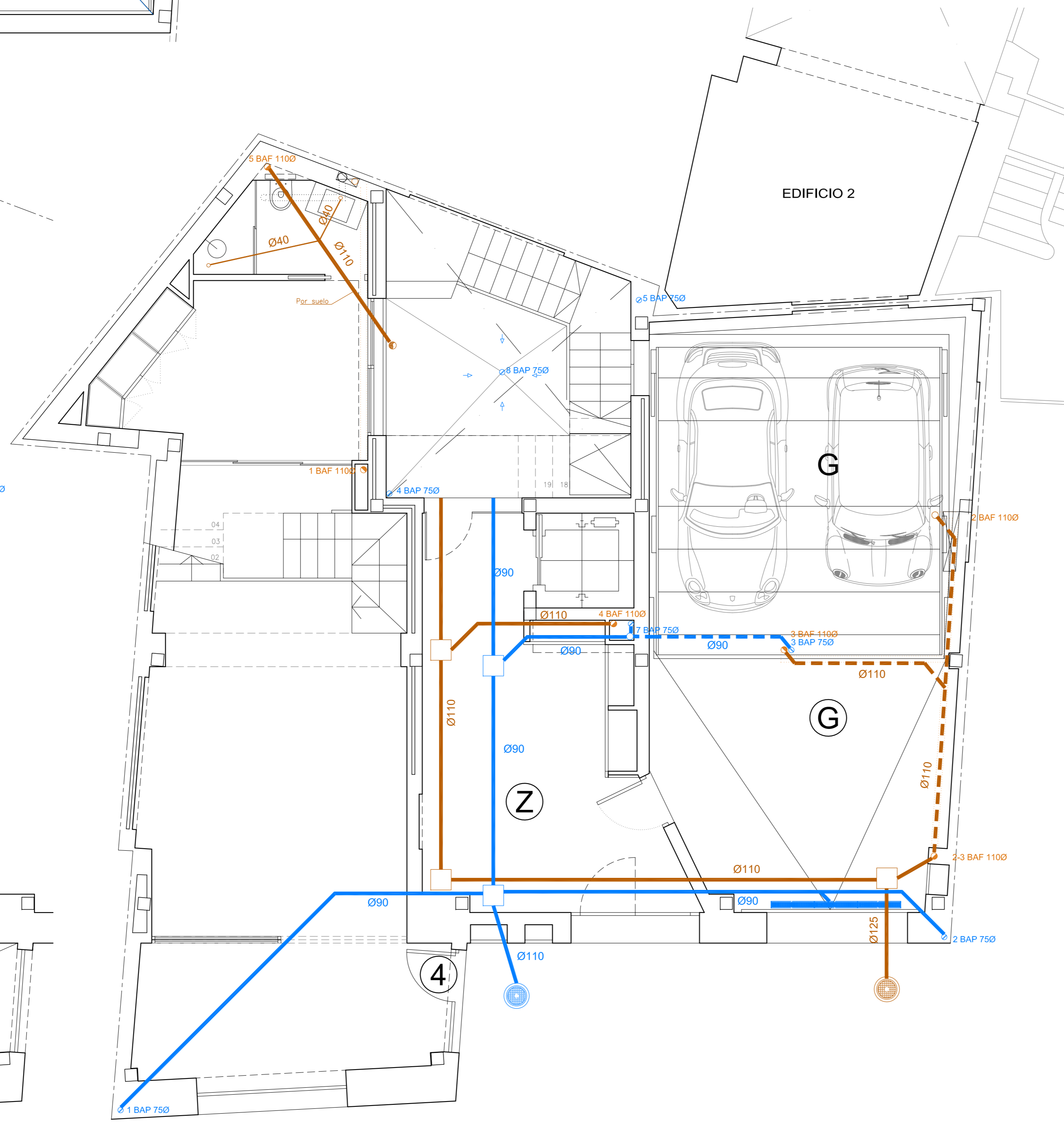
EDIFICIO 1 - PLANTA BAJA
