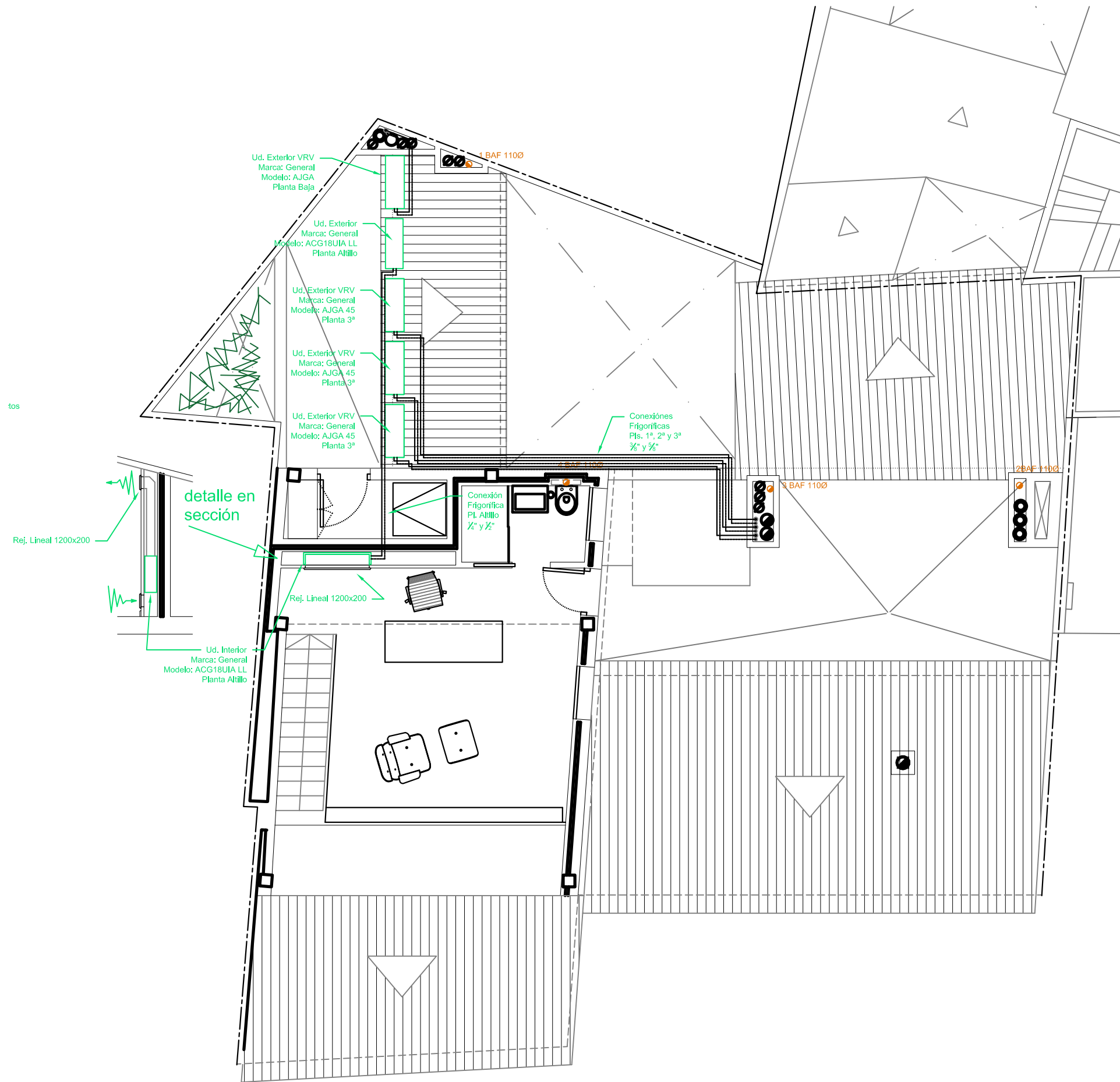
EDIFICIO 1_PLANTA ATILLO SUPERFICIE CONSTRUIDA 35.93 m2
